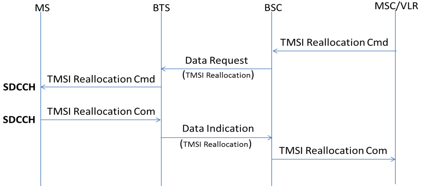
الشكل 6 - 8 - مرحلة تغيير هوية المشترك المؤقتة
