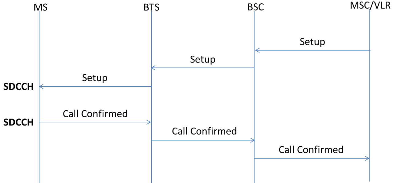
الشكل 6 - 10 - مرحلة تهيئة المكالمات
