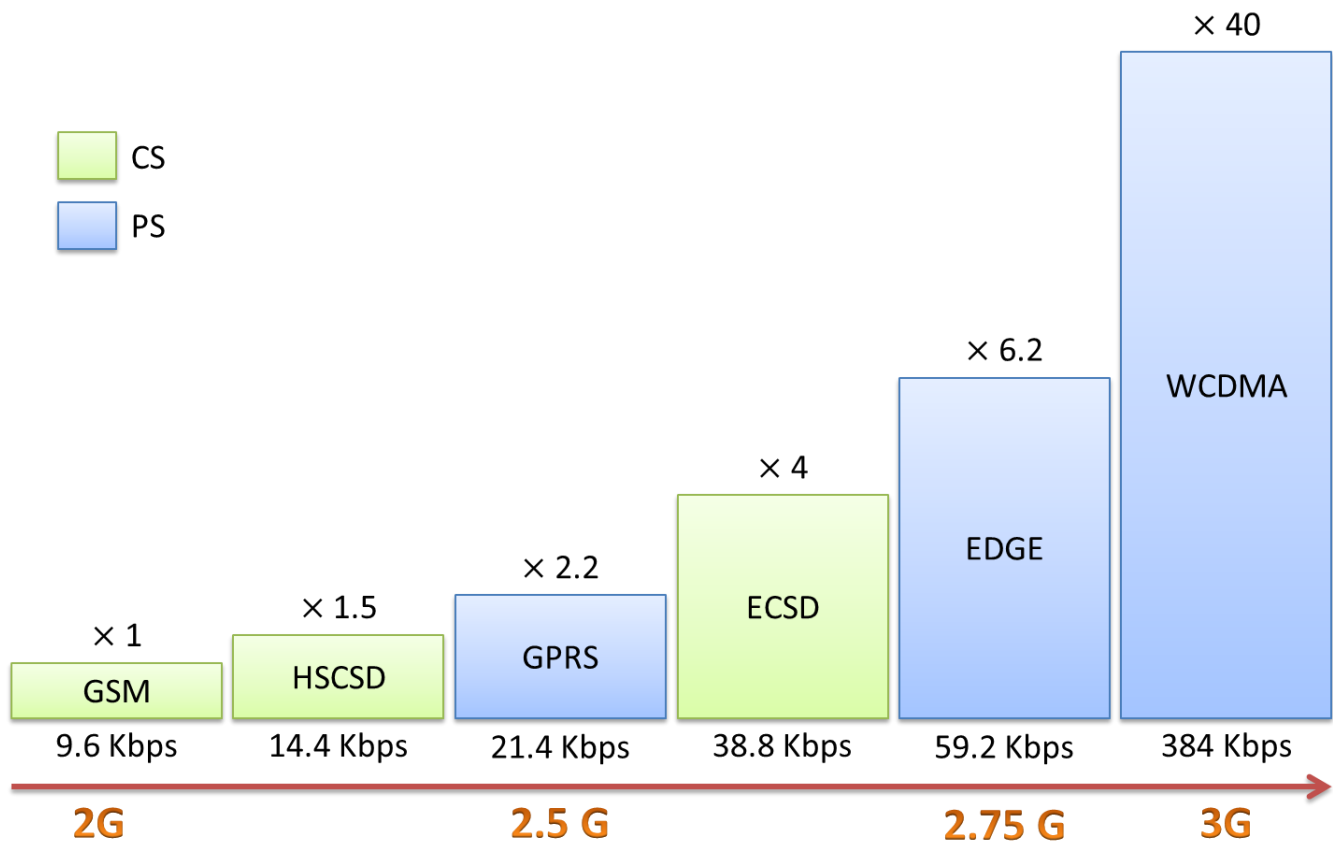
الشكل 7- 3 - مراحل تطور نظام الجيل الثاني إلى نظام الجيل الثالث
