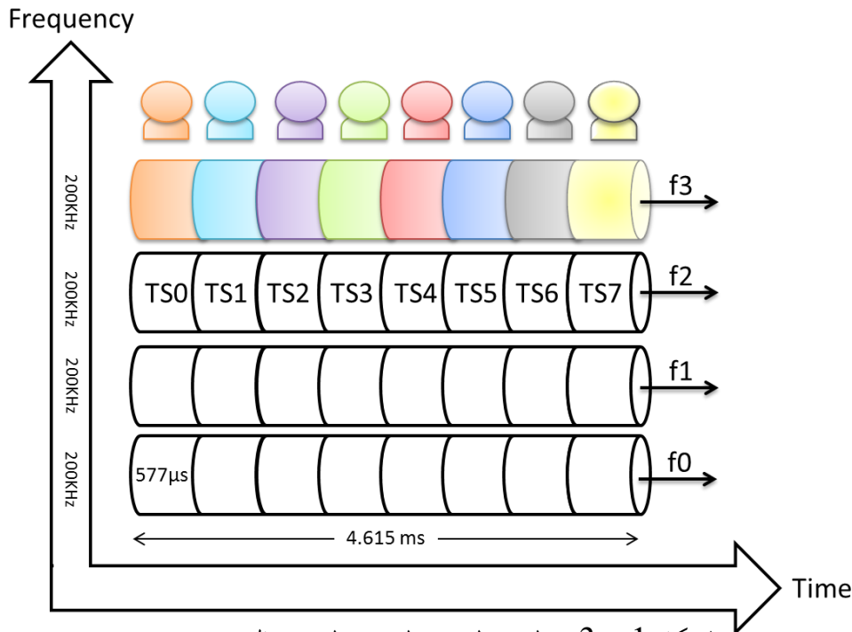
الشكل 1 - 3 - النفاذ المتعدد بالتقسيم الترددي والزمني
