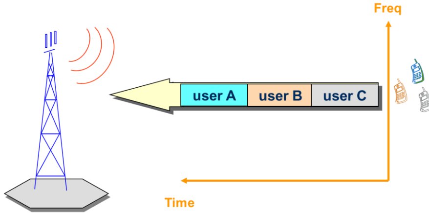
الشكل 1 - 2 - النفاذ المتعدد بالتقسيم الترددي
